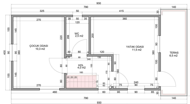
Üst Kat Planı
